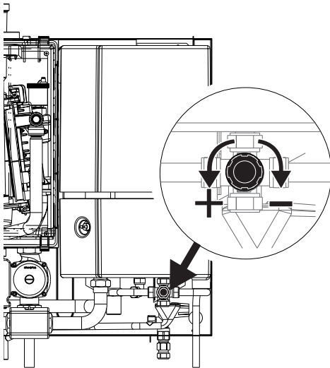
réglage mitigeur thermostatique figure 9.2.a
