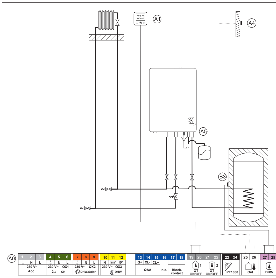
Direktheizkreis mit Warmwasserspeicher über Dreiwegeventil
