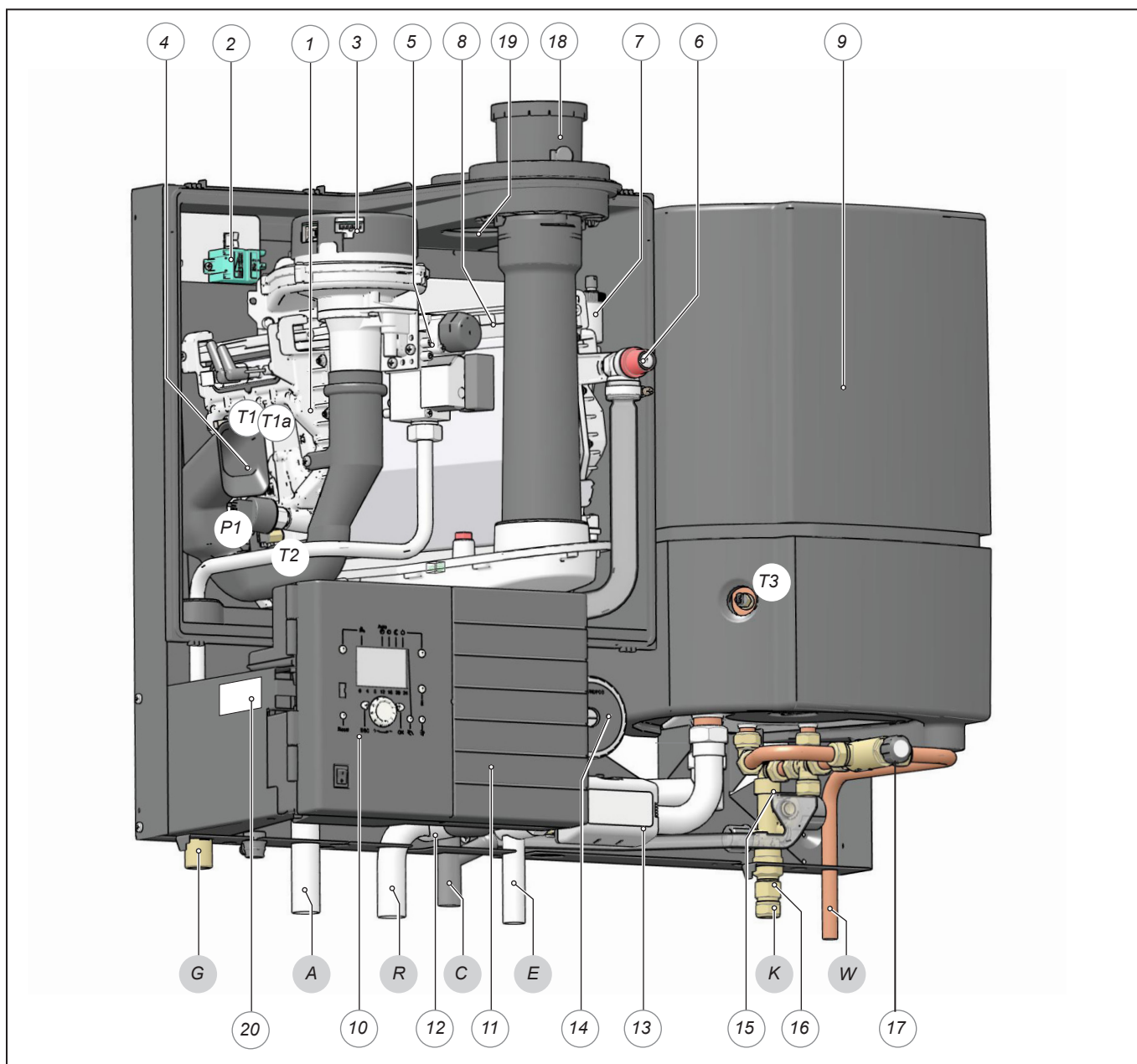
Kesselansicht ATAG QR-Kombikessel
