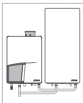
Kessel/Speicher-Kombination Q25SR + HQS110 Bild 7.1
