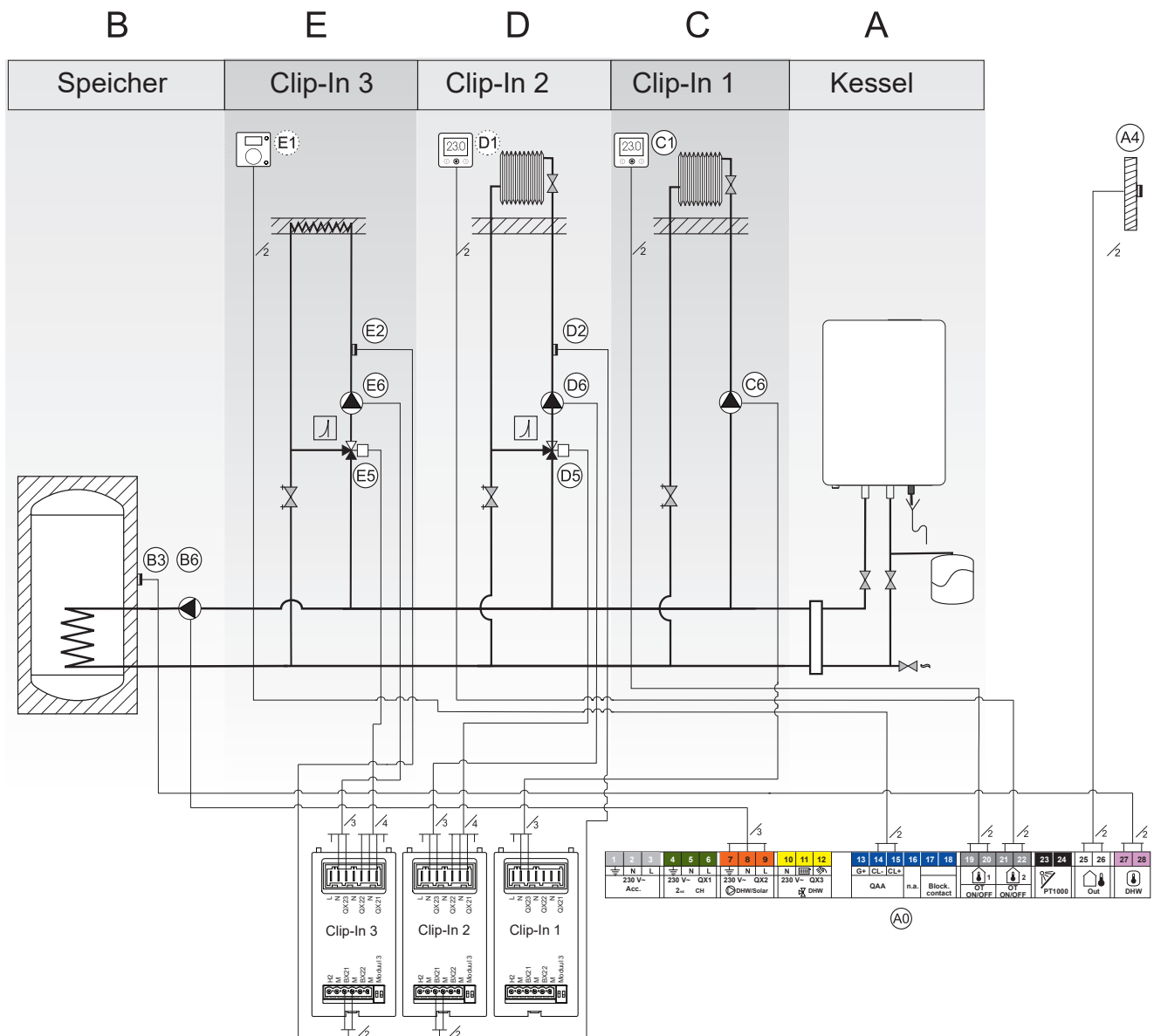
Direktheizkreis, zwei Mischerkreise, Speicherladepumpe
