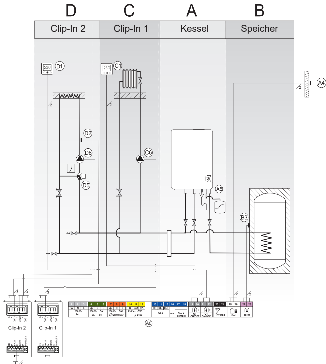
Direktheizkreis, Mischerkreis, Warmwasserspeicher über Dreiwegeventil
