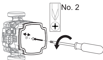
Deblockierung Kesselpumpe
