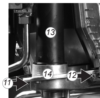
Kondensatwanne Bild 10.3.i
