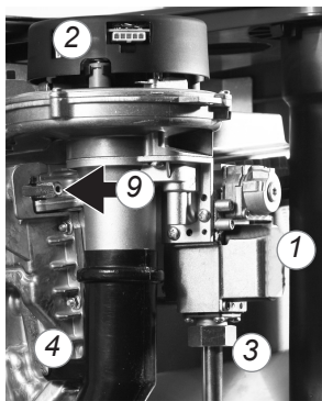
Ventilator und Gasventil Bild 10.3.c
