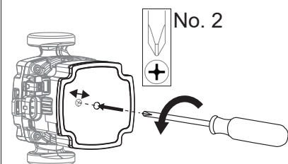
Deblockierung Pumpe
