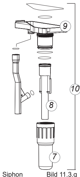
Siphon Bild 11.3.g
