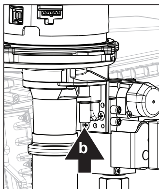
Einstellschraube O 2 / CO 2 Bild 10.5.b
