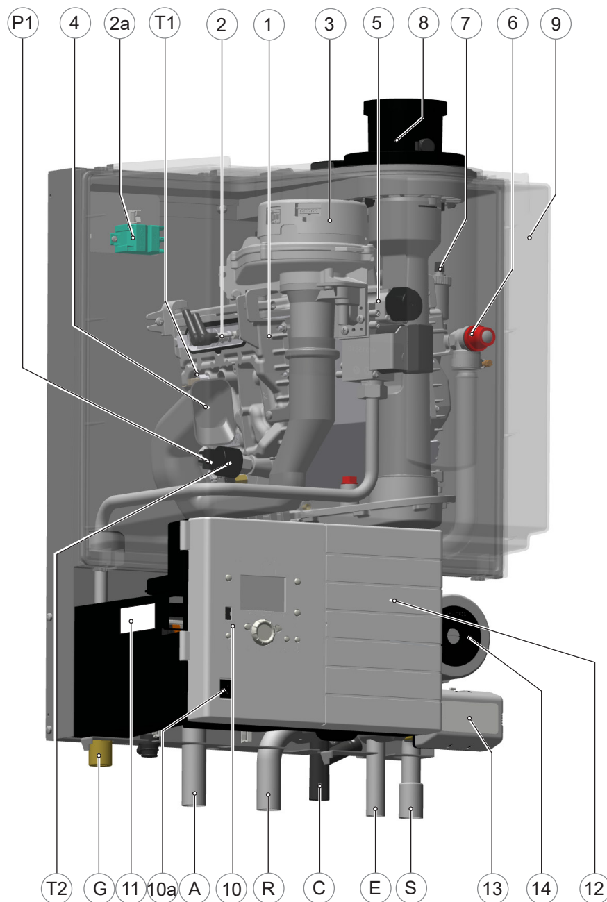
Schematische Darstellung ATAG QR-Solar Kessel
