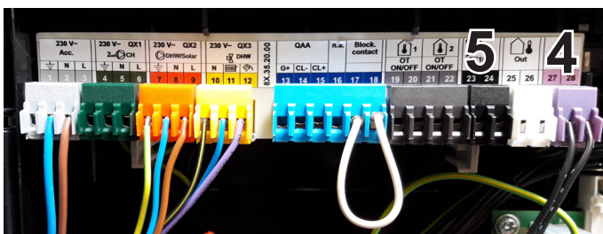
Anschlussklemmen ATAG QR-Solar-Kessel
