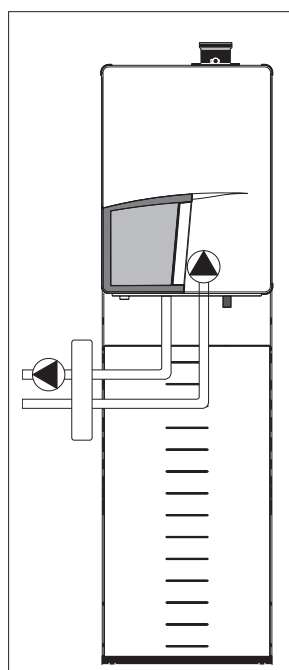
Externe Heizungspumpe mit offenem Verteiler
