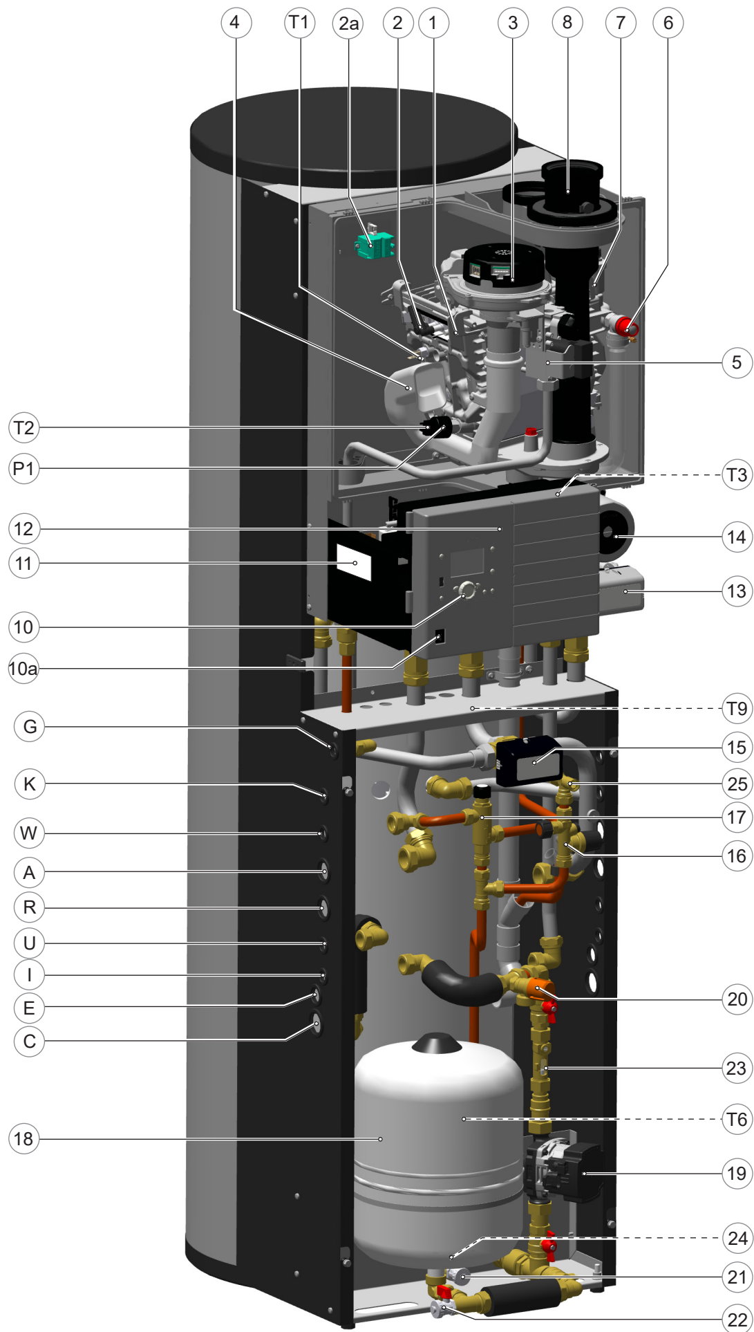
Schematische Darstellung ATAG QR-Solar (Q25SCR200N)
