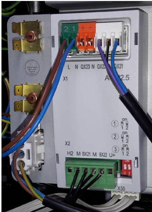
Solarmodul
