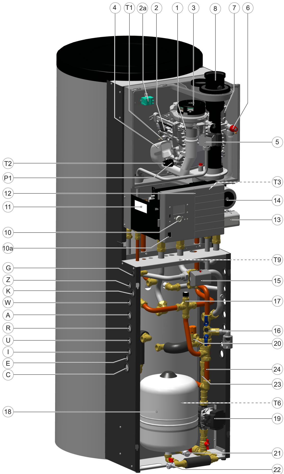
Schematische Darstellung ATAG QR-Solar (Q38SCR380N)
