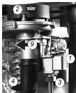
Ventilator und Gasventil
