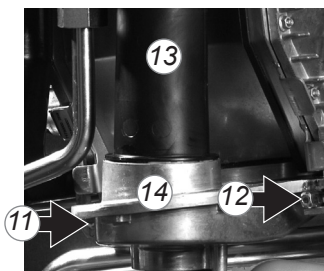
Kondensatwanne Bild 11.3.h
