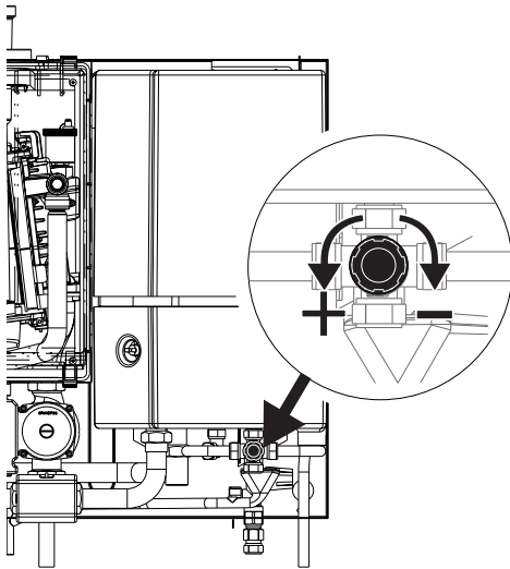
instellen thermostatisch mengventiel figuur 9.2.a
