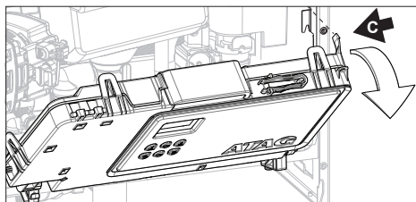
Kantelen bedieningsunit
