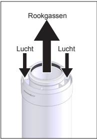
Stromingsrichting concentrisch Figuur 8.8.2.b
