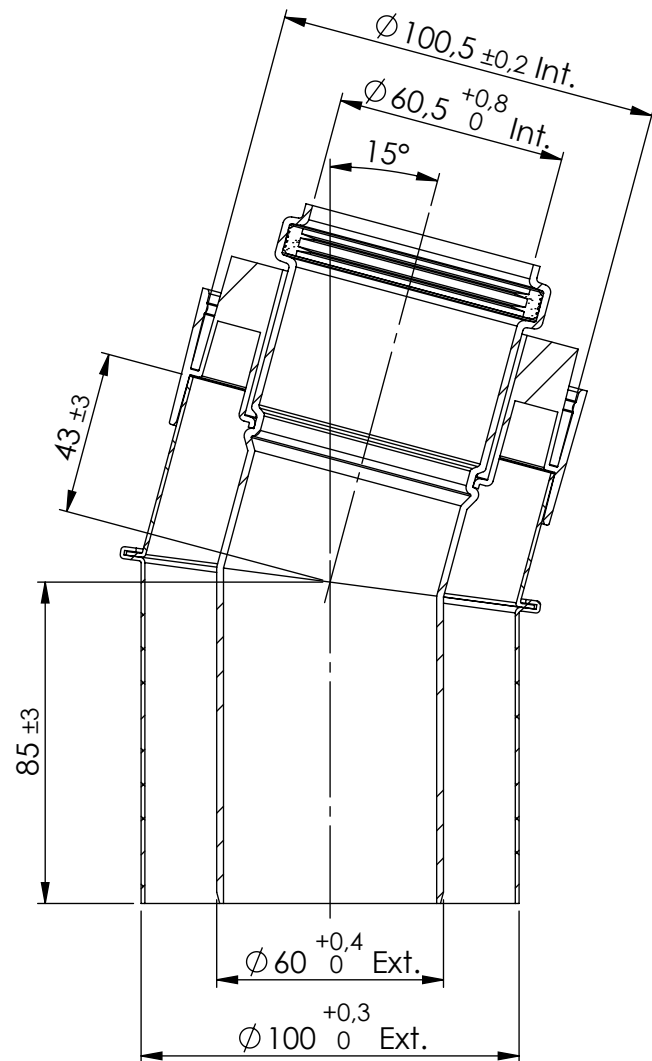
SECTION A-A
