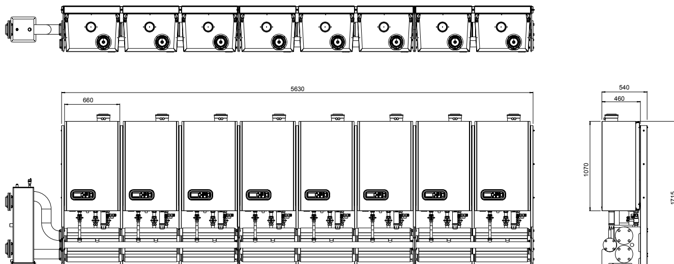
ATAG XL 8 ketels vrijstaand in lijn
