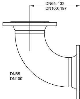
Afmetingen bocht DN65 en DN100
