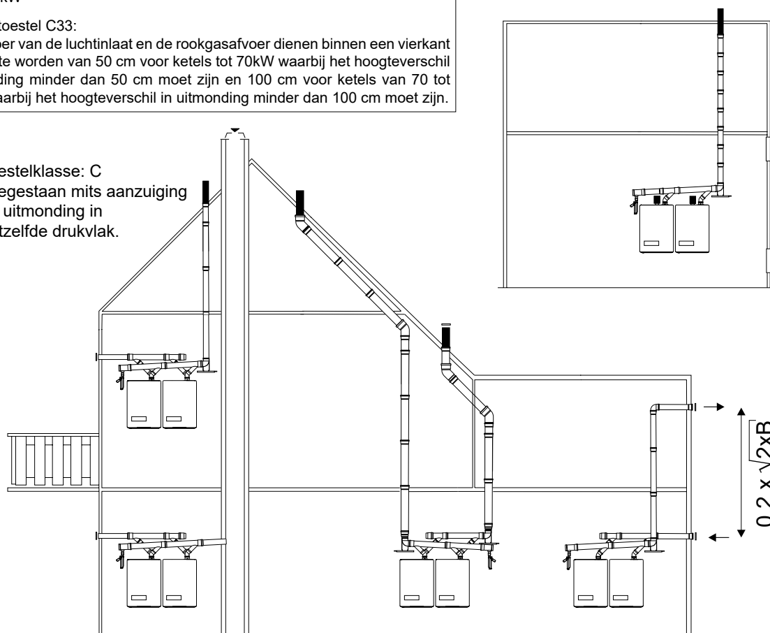
Mogelijkheden uitmondungen collectieve rookgasafvoer
