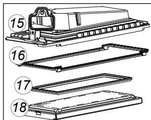
Bovenbak, brander en afdichtingen Figuur 13.4.d
