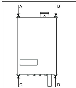
Mantel verwijderen Figuur 13.4.a
