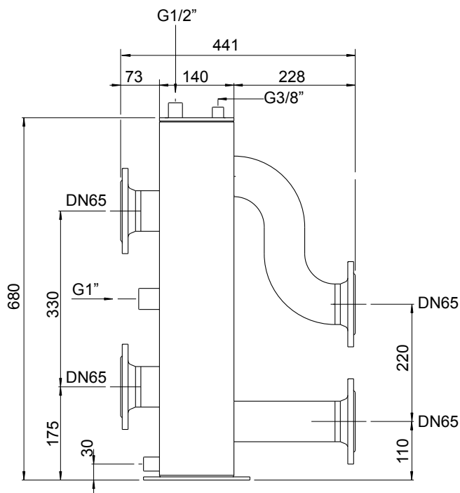
Afmetingen open verdeler DN65 tot 452kW
