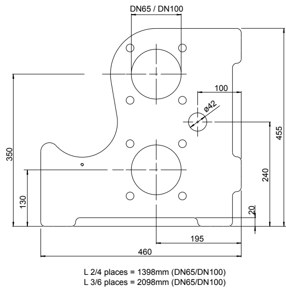
Afmetingen verzamelleidingen
