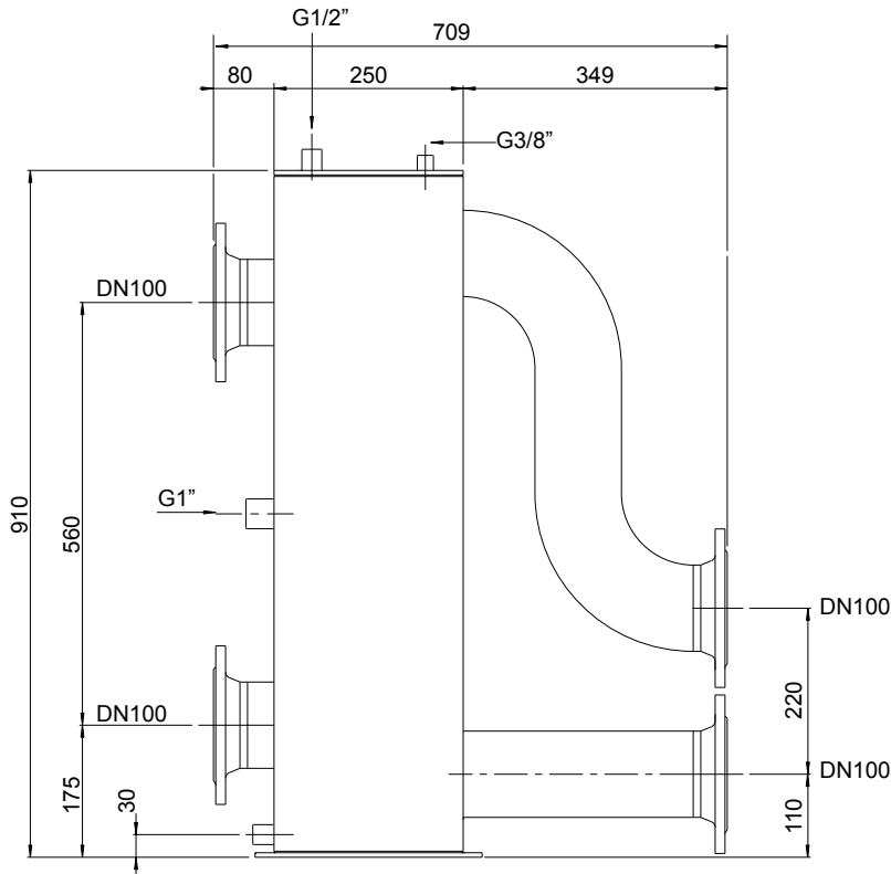
Afmetingen open verdeler DN100 tot 960kW
