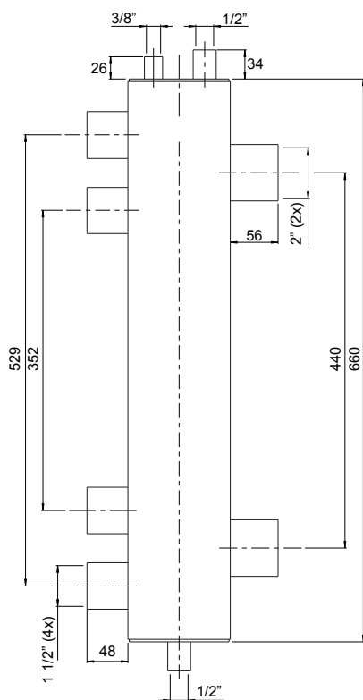
XL 1 ketel, vrijstaand
