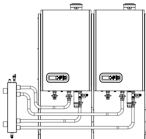
XL 2 ketels, vrijstaand
