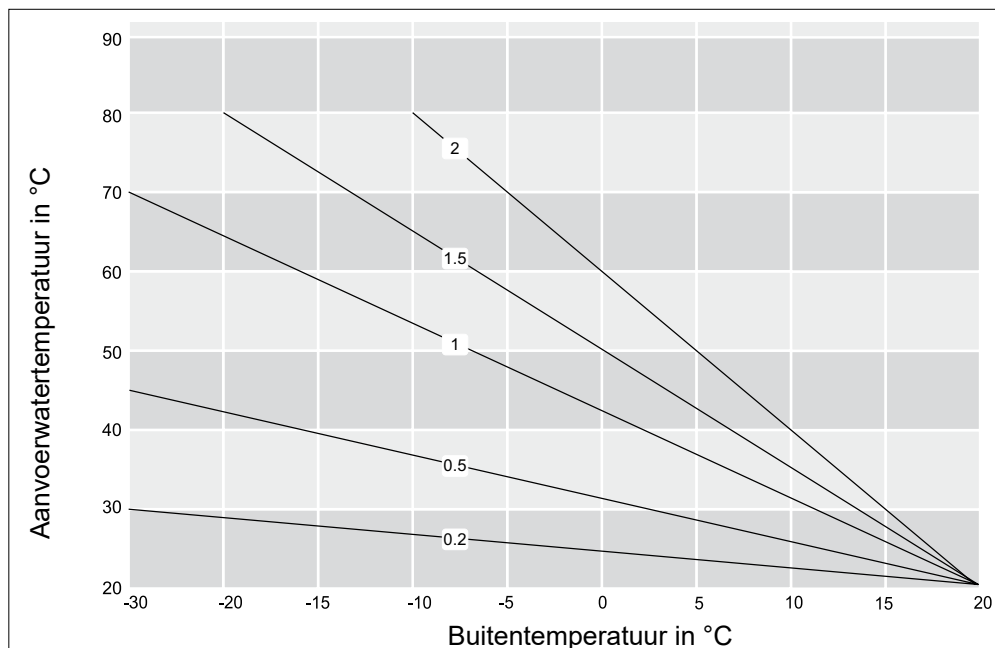
Stooklijningrafiek (K-factor)
