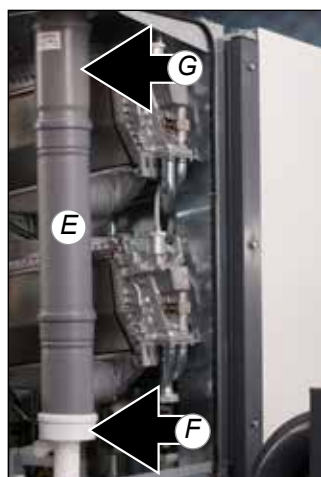
Rookgasafvoerpijp uitbouwen Figuur 13.4.b
