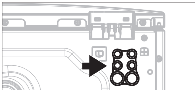
Doorvoer bekabeling onderzijde ketel
