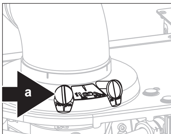
a Meetpunt voor rookgasanalyse
