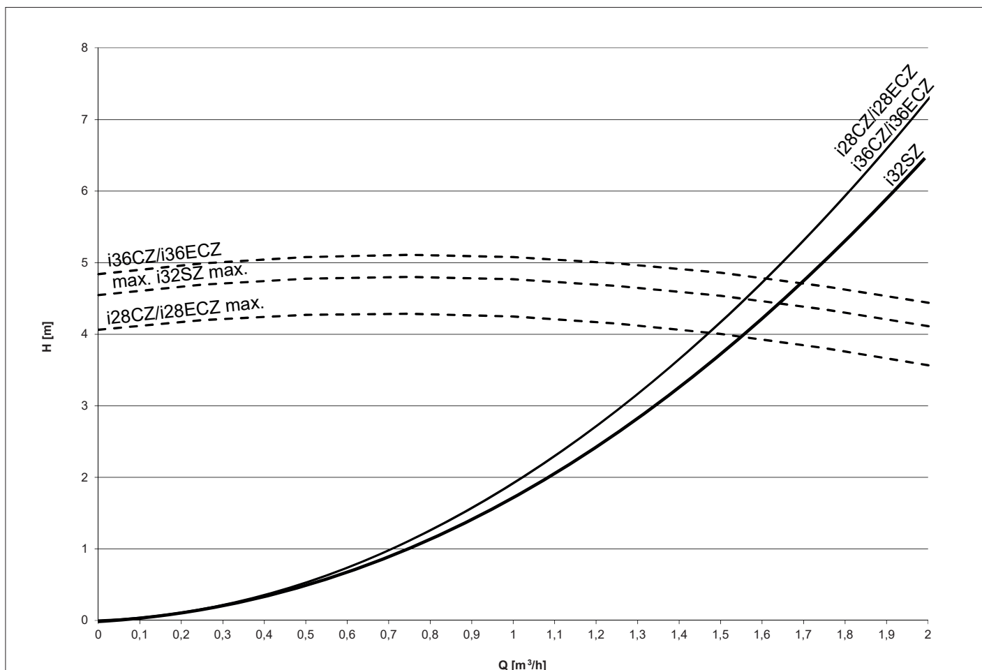
Pompkarakteristiek
