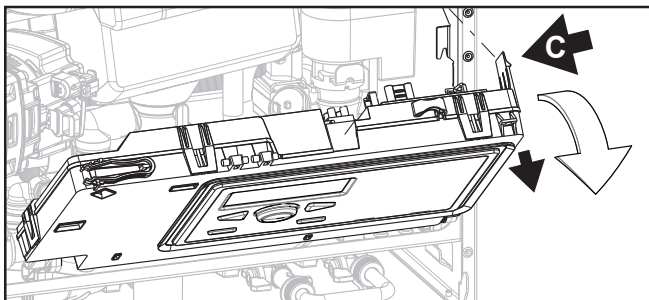
Openen besturingskast
