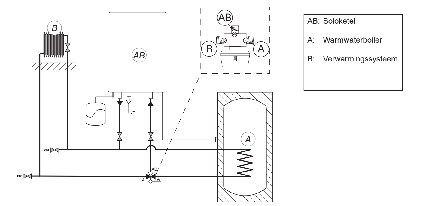
Hydraulisch schema met externe boiler
