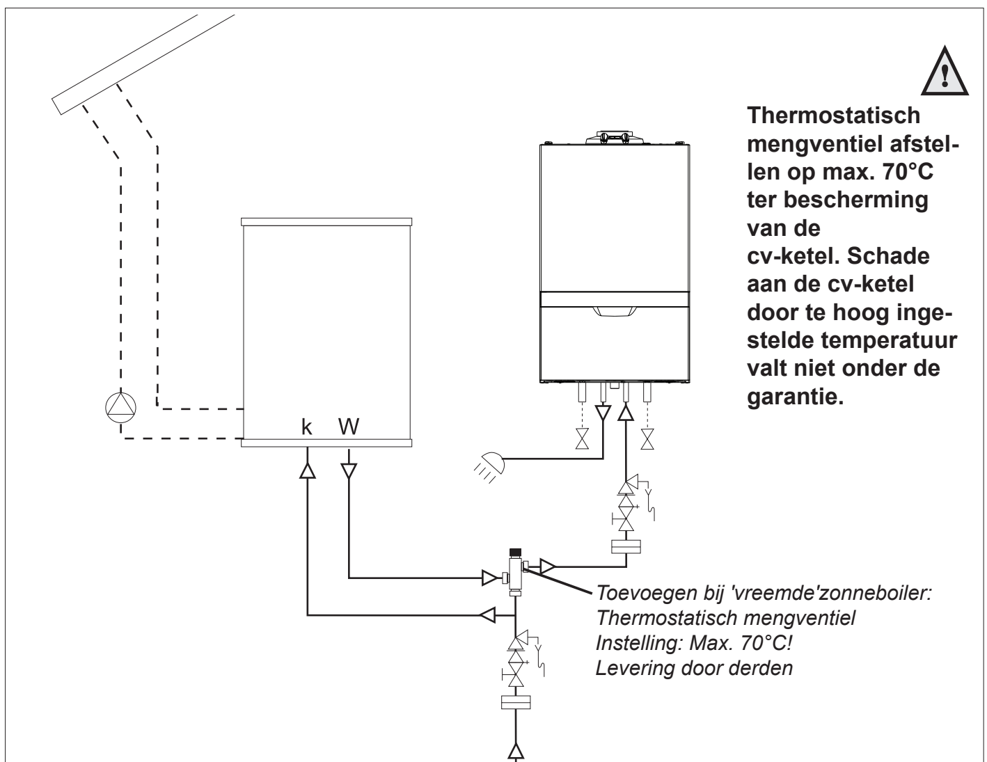
ATAG i Zone-Serie combiketel met zonneboiler
