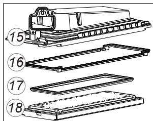
Bovenbak, brander en afdichtingen Figuur 12.2.f
