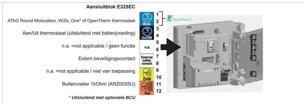
aansluitblok
