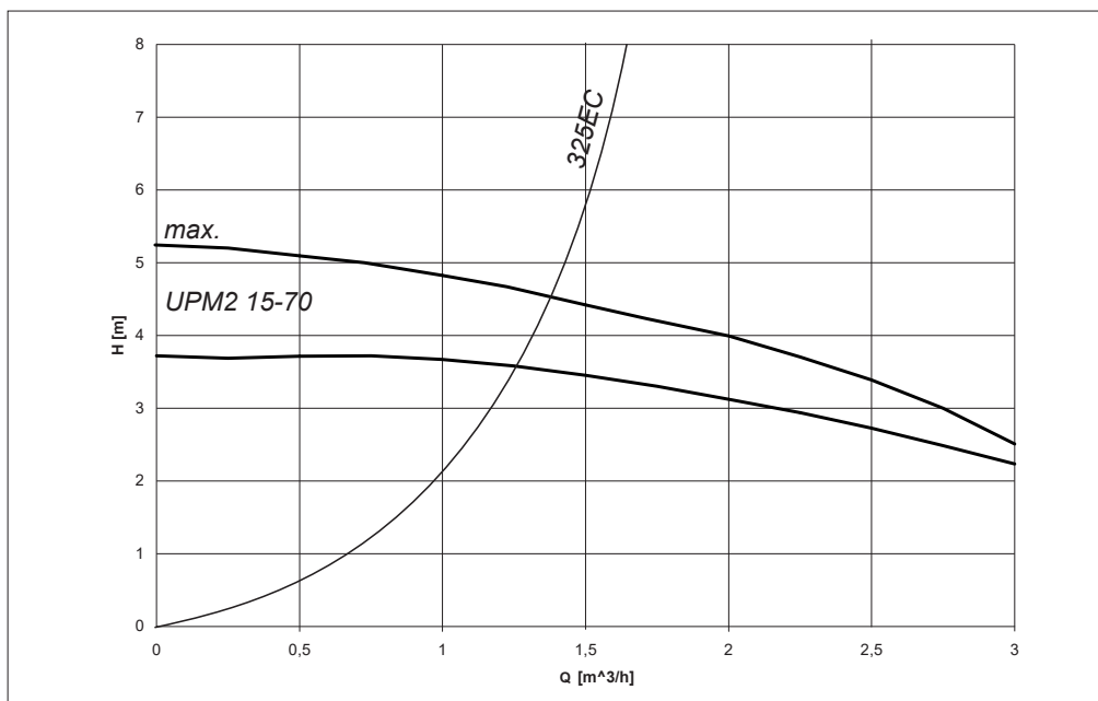
Pompkarakteristiek
