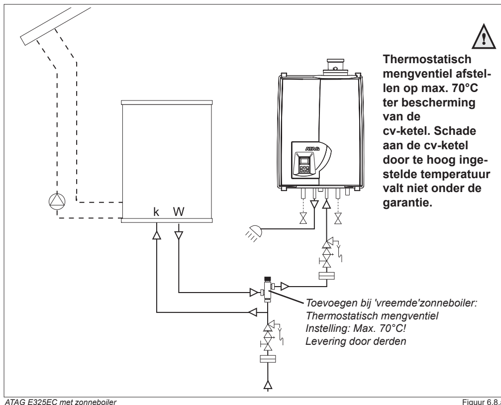
Figuur 6.8.a geeft een voorbeeldaansluitschema weer van de ATAG E325EC met een standaard zonneboiler.
