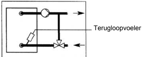
Geregelde toevoerbijmenging met meng- of mengklep
