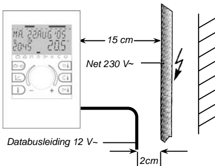
Afb. 1: Minimumafstanden bij de elektrische installatie
