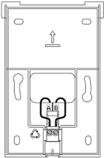
Aansluitsokkel (bovendeel verwijderd)
